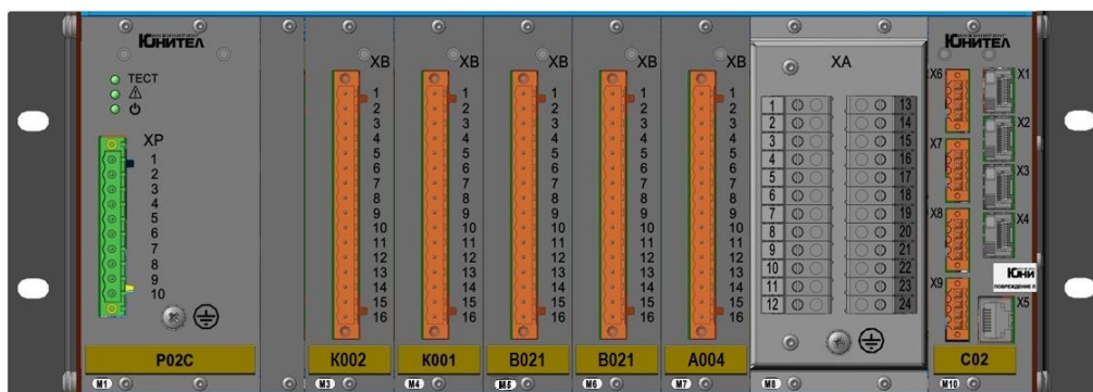
Рисунок 1.1 – Вид устройства ЮНИТ-М314-АРНТ с размещением плат по слотам (для ПС со смешанной или I архитектурой, исполнение I)
